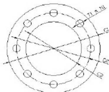
Верхний фланец (горизонтальный разрез)
