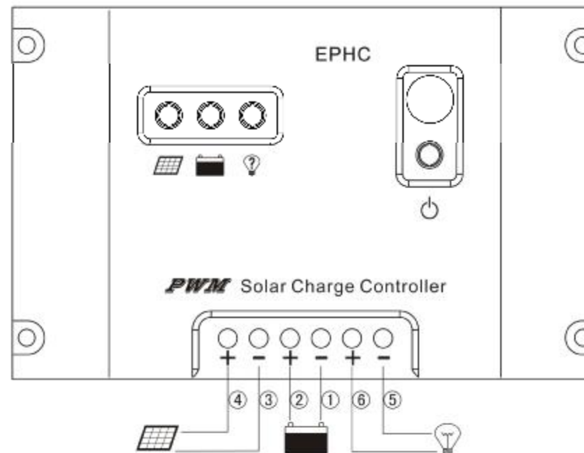
Рис.1 Последовательность подключения оборудования к контроллеру
