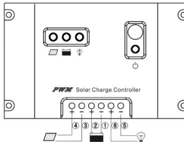
Рис.1 Последовательность подключения оборудования к контроллеру
